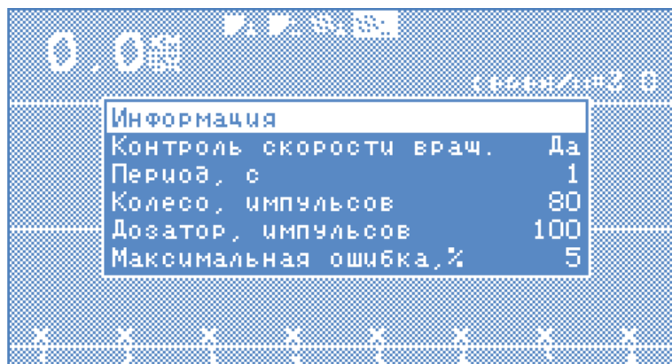
Рисунок 8 Параметры дозатора
