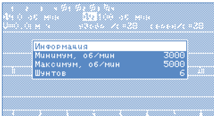
Рисунок 11 Параметры вентилятора
