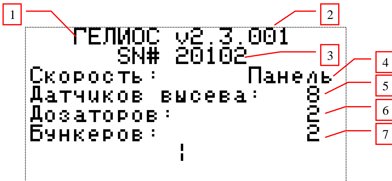
Рисунок 2 Экран конфигурации
