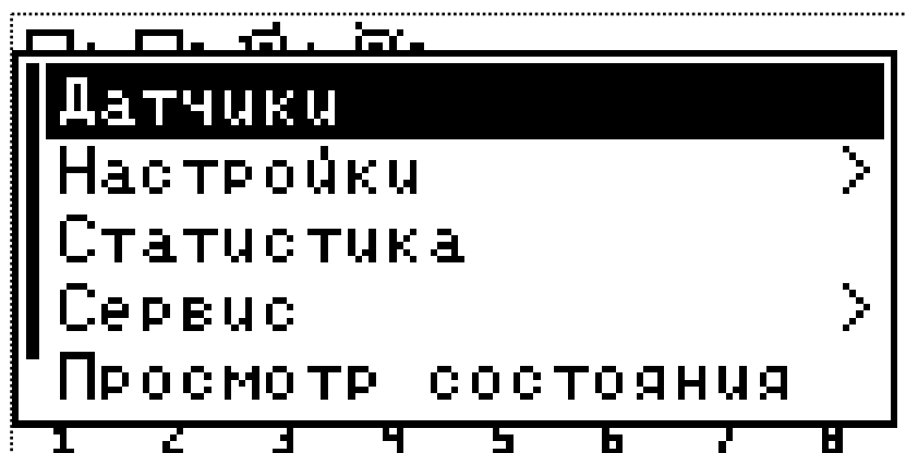
Рисунок 11 Главное меню
