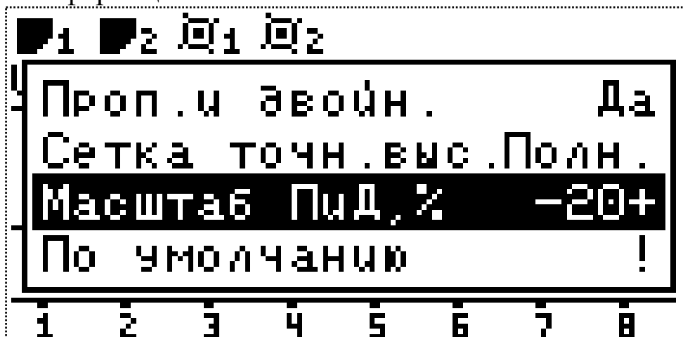
Рисунок 14 Параметры диаграммы
